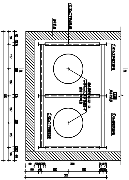
1#泵站底板面平面布置图 1:33
